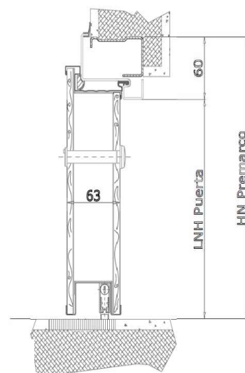
Sección vertical:
