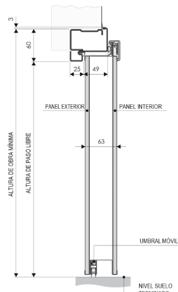
Sección vertical:
