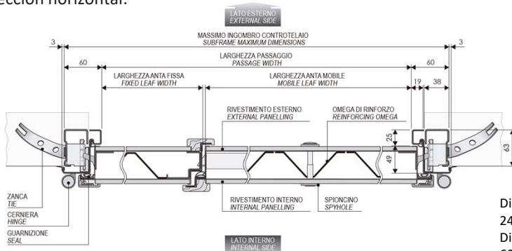
Sección horizontal:
